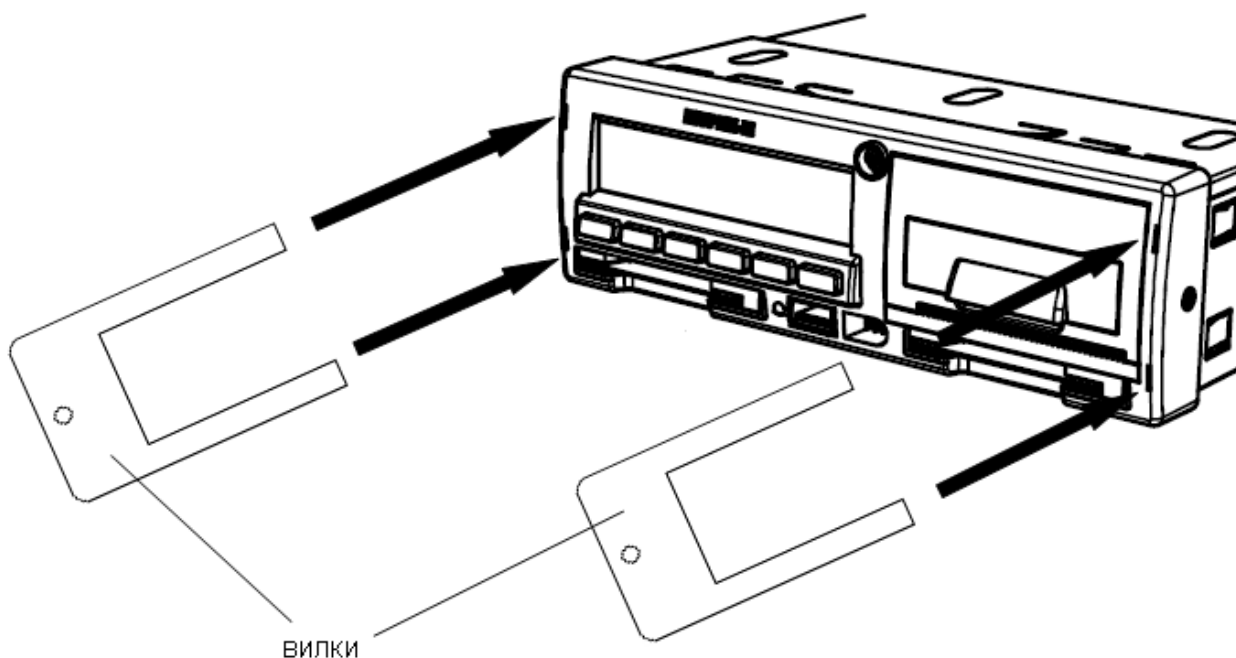
Рисунок 4 – Извлечение тахографа
