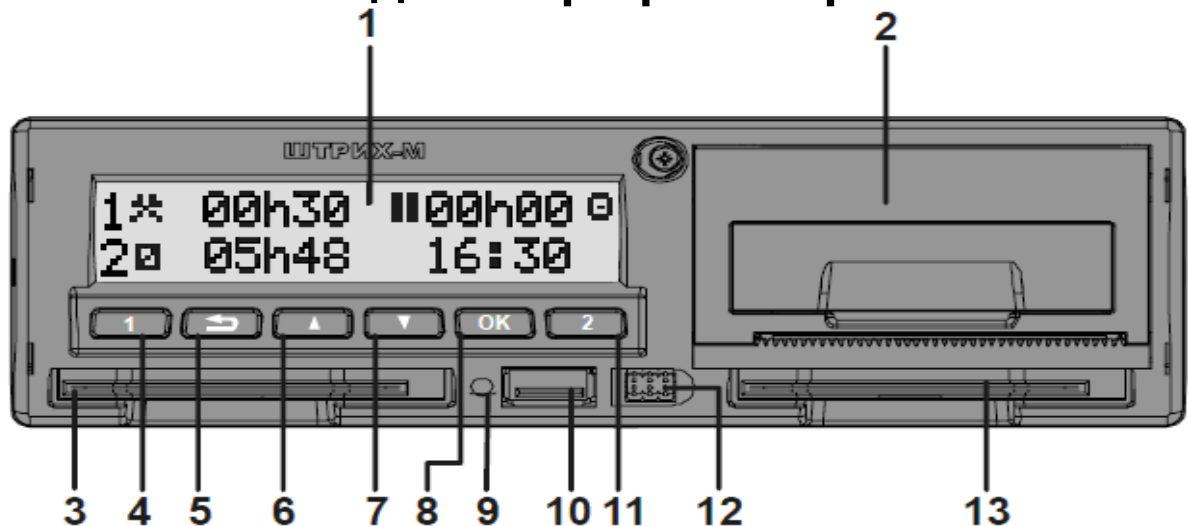
Рисунок 2 – Внешний вид передней панели тахографа
