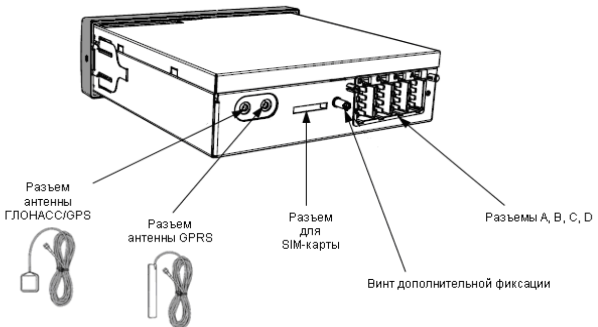
Рисунок 3 – Внешний вид задней панели тахографа
